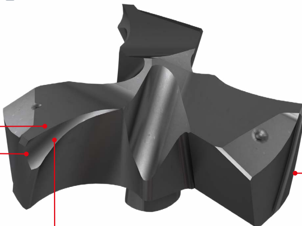
1 Flachbohrkopf
